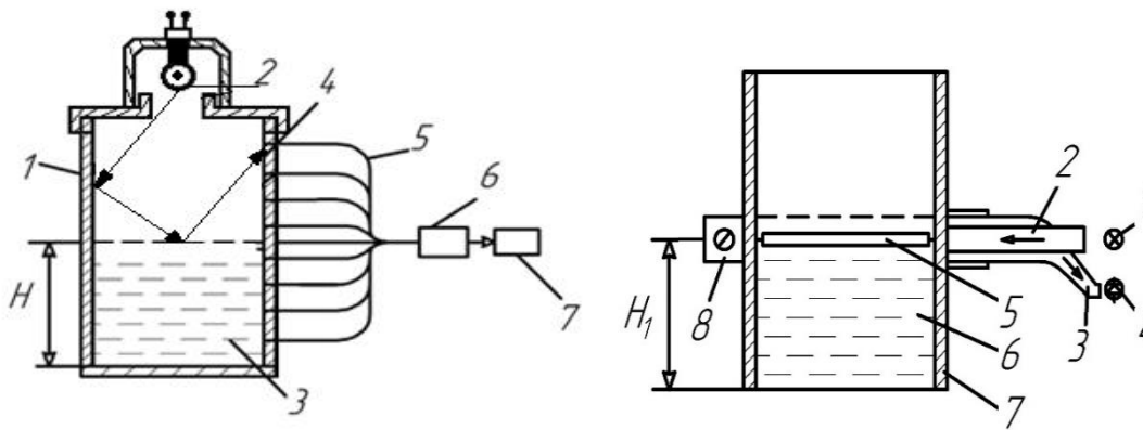
Рис.2. Физические модели ОДПВ.
