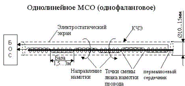
Рис. 1. Однолинейное магнитометрическое средство обнаружения (однофланговое)
