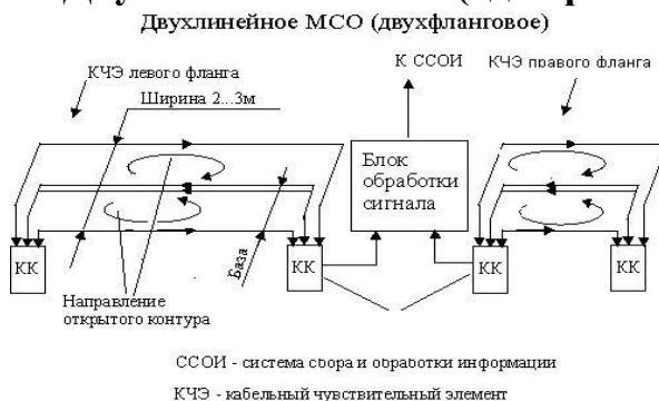
Рис. 2б. Двухлинейное МСО (двухфланговое)
