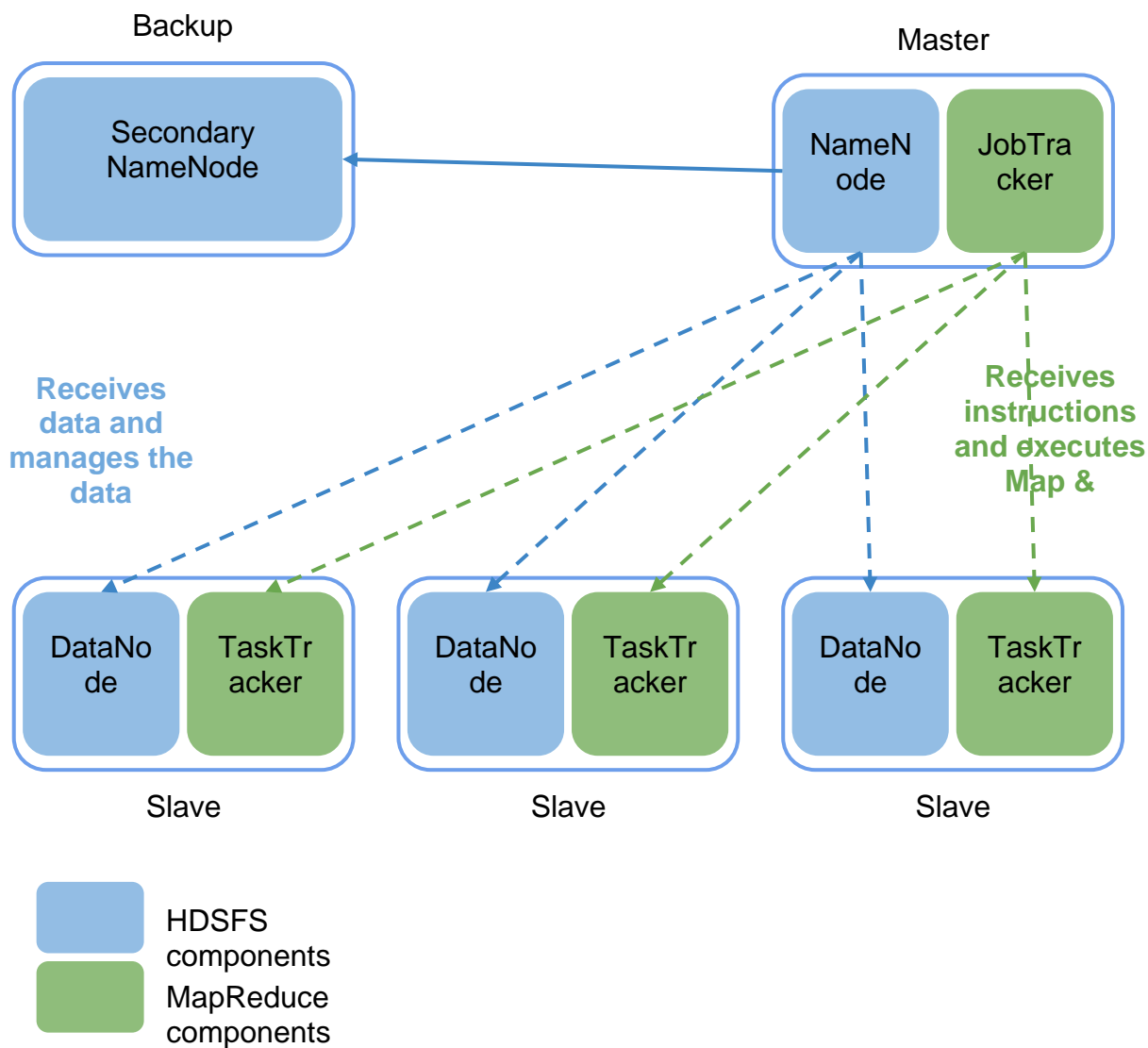
Rasm 4. Umumiy arxitektura
